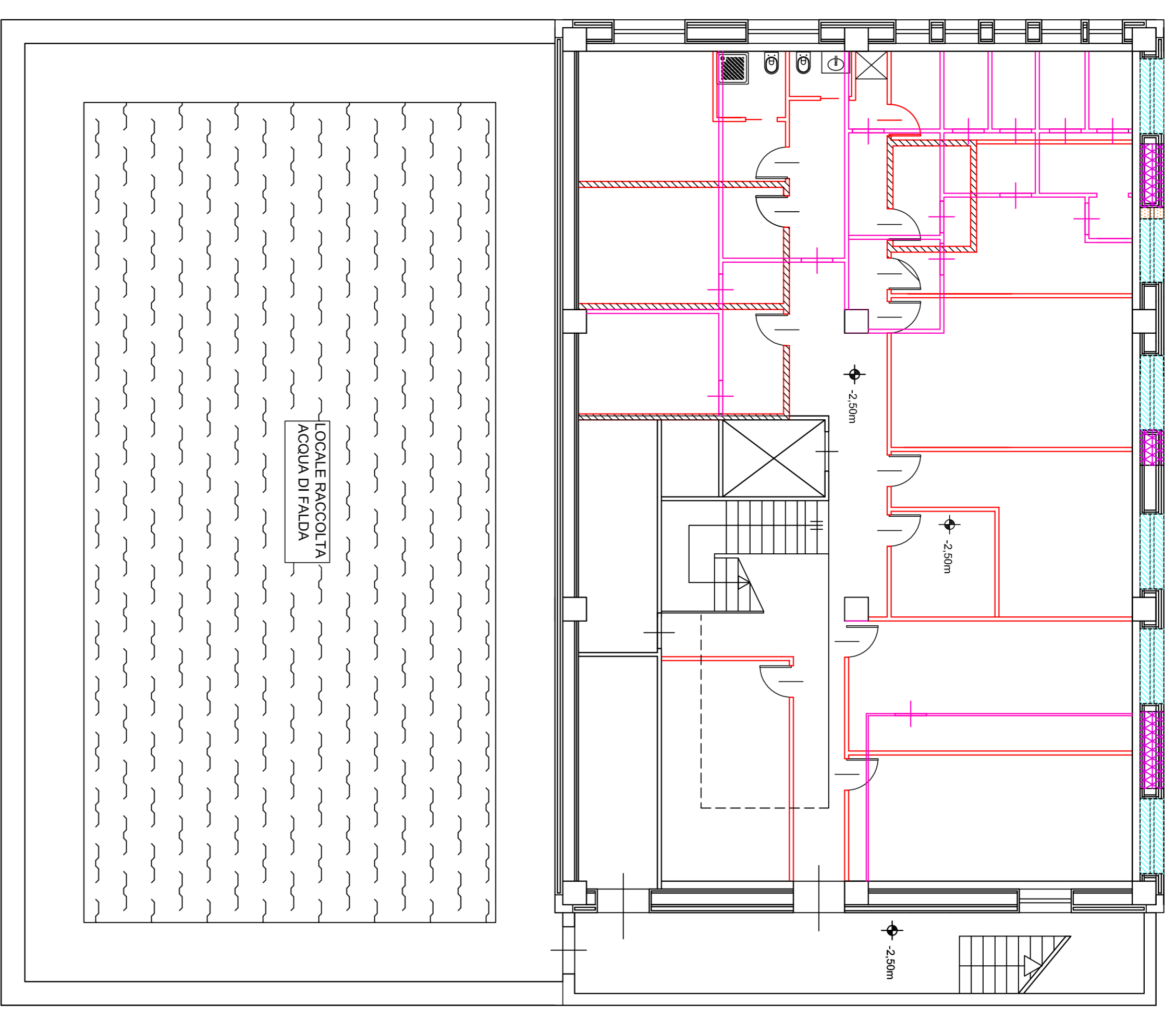
PIANTA PIANO SEMINTERATO
