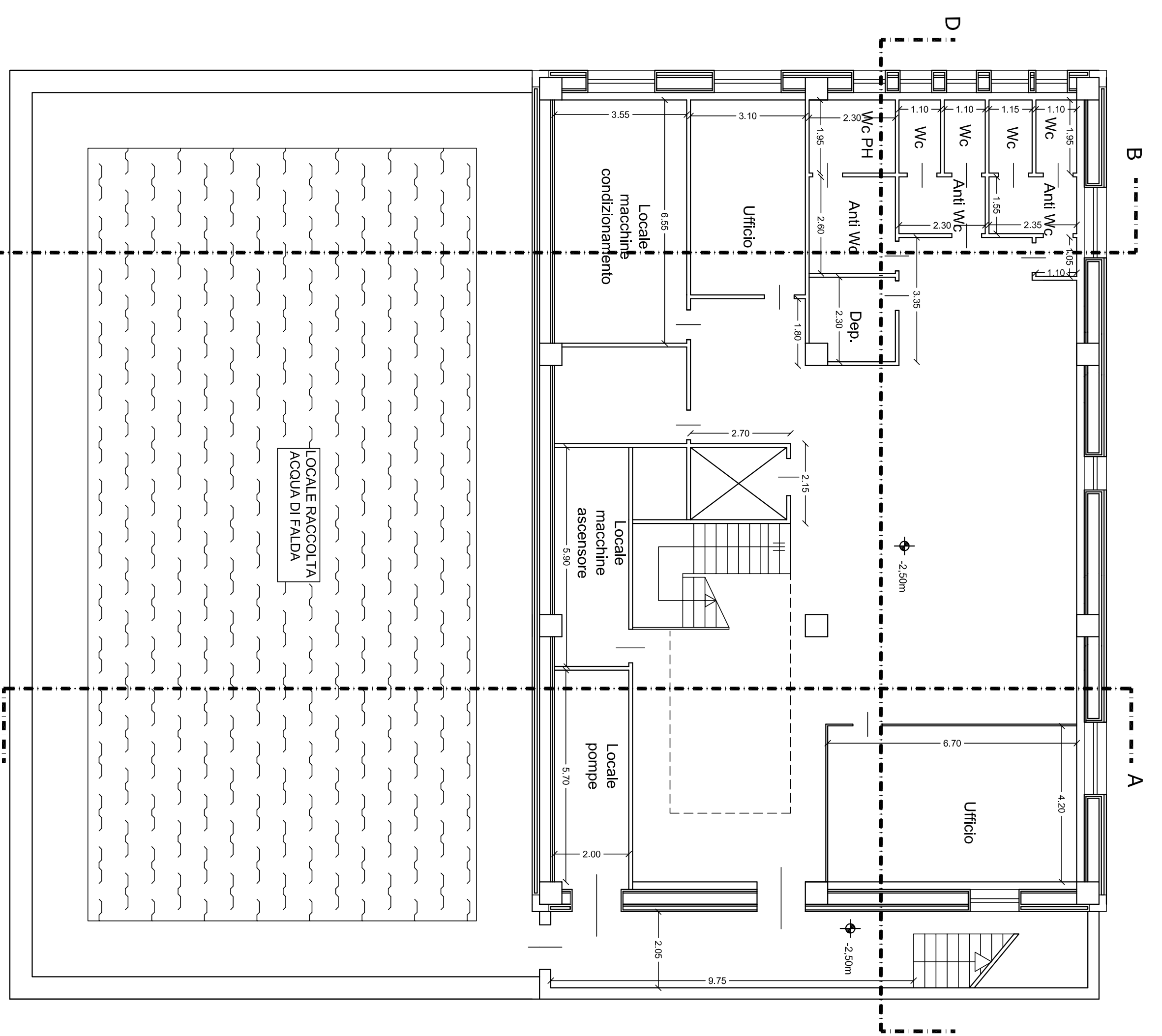
PIANTA PIANO SEMINTERATO
